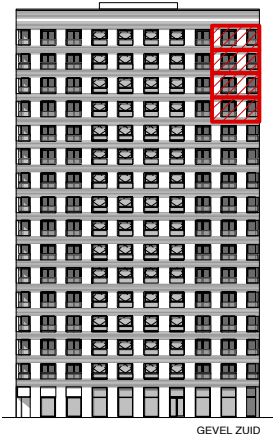
GEVEL ZUID
